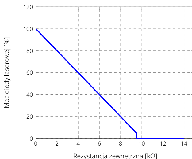
Moc diody laserowej vs. rezystancja zewnętrzna
