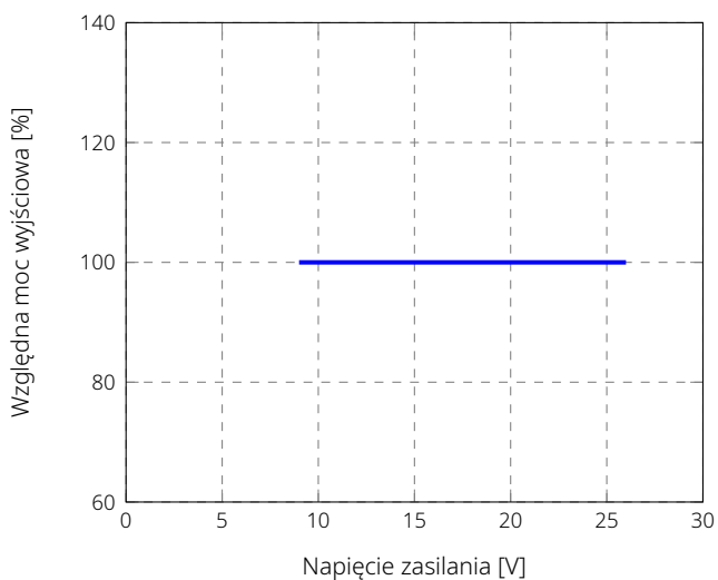
LWPRO-450-1000-MM Względna moc wyjściowa vs. napięcie zasilania
