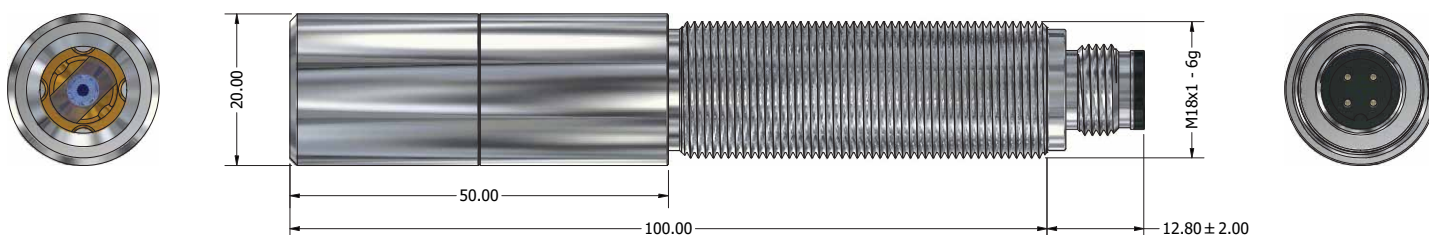
Wykonywany na zamówienie wariant -M18x1-M12/4P z 4-pinowym złączem M12 i gwintem zewnętrznym M18x1
