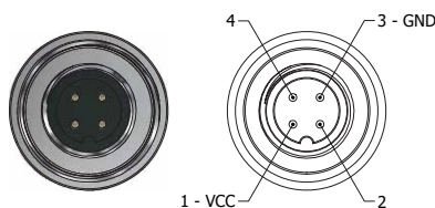
Złącze zasilające M12 4-pin
