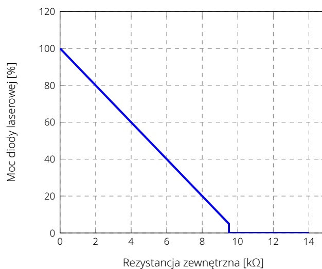
Moc diody laserowej vs. rezystancja zewnętrzna
